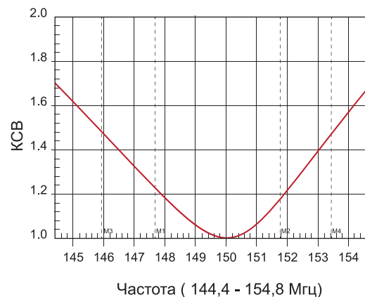
Стандартное КСВ X-130 VHF
